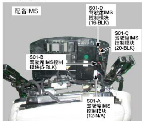
234. 驾驶席座椅
