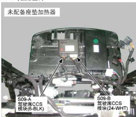
233. 驾驶席座椅
